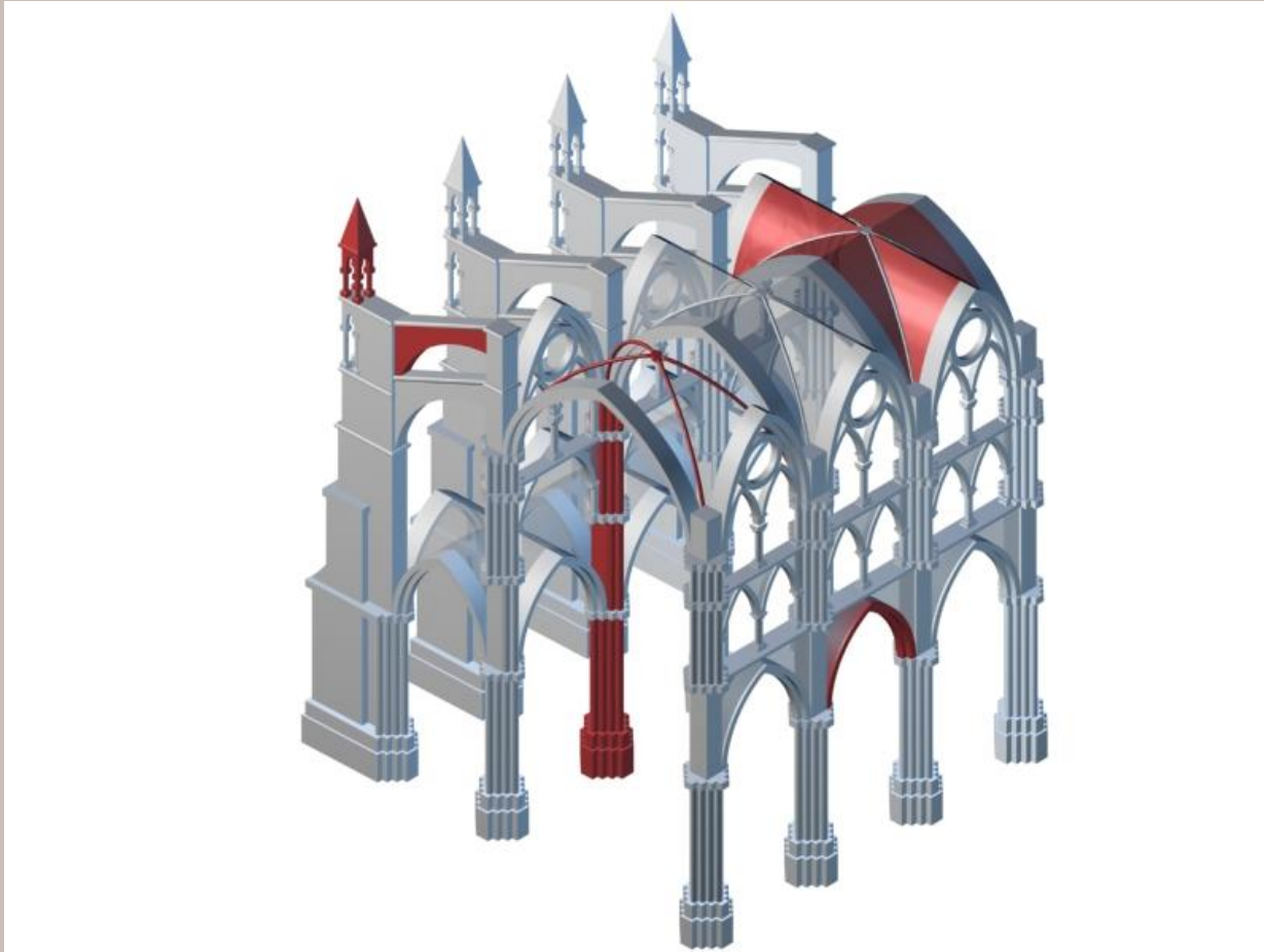
Obr. 4 Vnější a vnitřní opěrný systém
