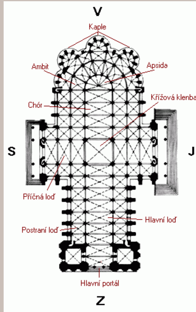
Obr. 3 Půdorys katedrály
